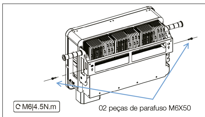
Figura 5.15: Parafusos inversor/suporte.
