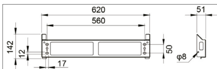
Figura 5.7: Medidas suporte de parede.
