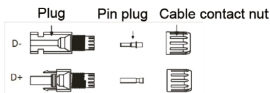
Figura 6.16: Peças conector CC.
