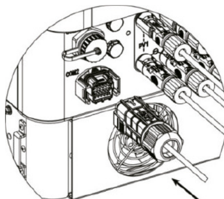
Figura 6.24: Fixação COM.
